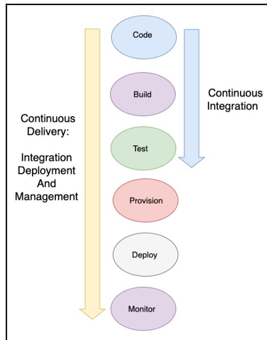
CI/CD
