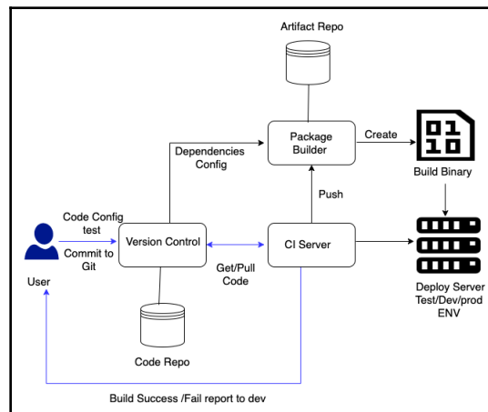
CI/CD for DevOps
