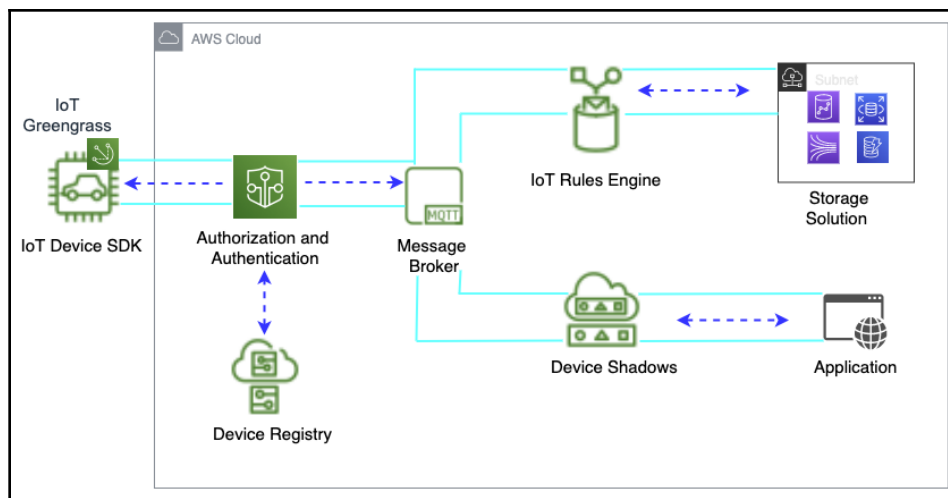
AWS IoT
